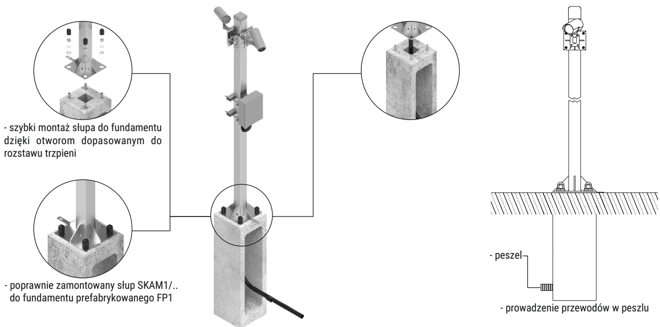
Przykład zastosowania fundamentu prefabrykowanego FP1
