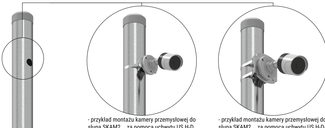
Przykład zastosowania uchwytów US H-D i US H-D-1
