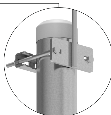
Przykład zastosowania iglicy odgromowej IODG
