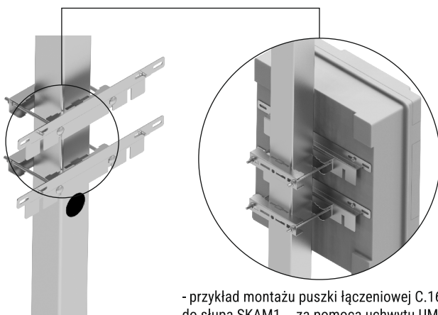
Przykład zastosowania uchwytu uniwersalnego UMB1
